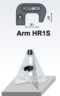
Ablagegeständer Art.-Nr.: 054158
