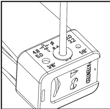
Medidor do diâmetro do rebite
