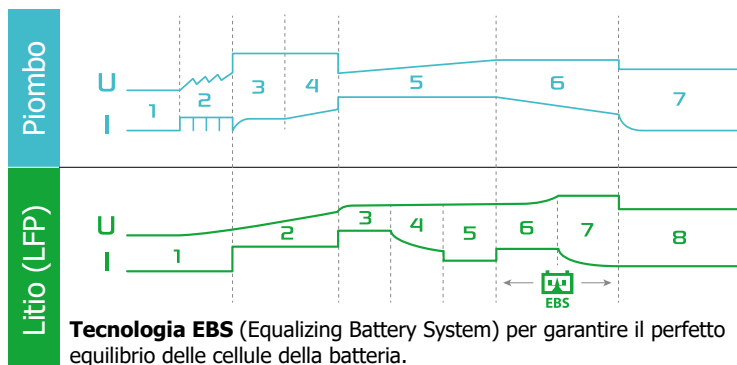
Curva di carica specifica in 7 tappe senza sorveglianza.
